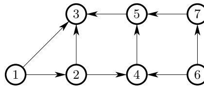
Figura 3.33 Digrafo de una matriz triangular
